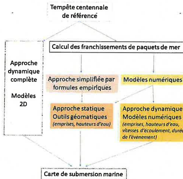
Figure 1 : Synthèse des 3 approches envisageables pour l'évaluation des franchissements de paquets de mer et la cartographie de la submersion marine.
